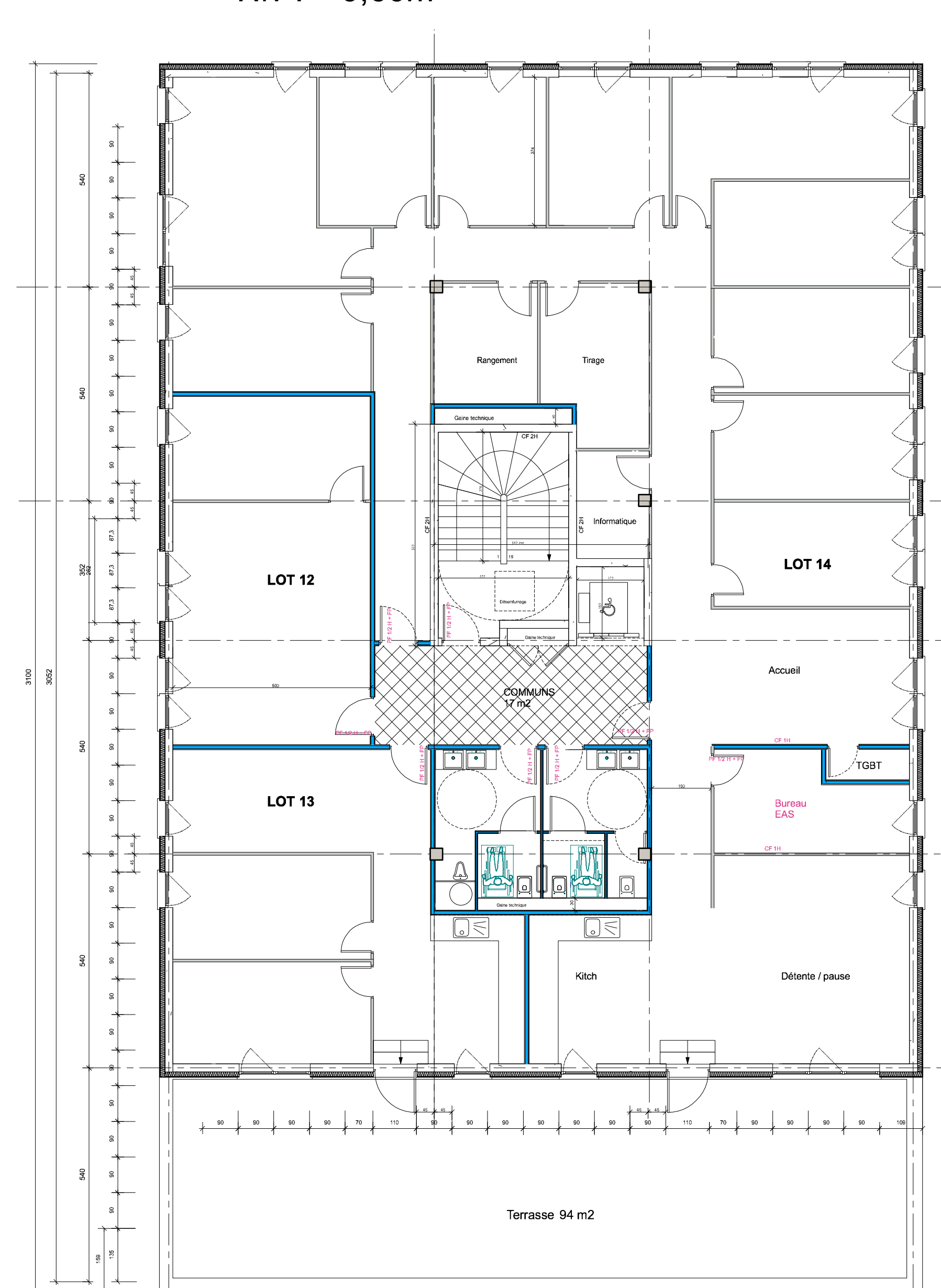
Plan étage +3 Niv : + 9,60m
