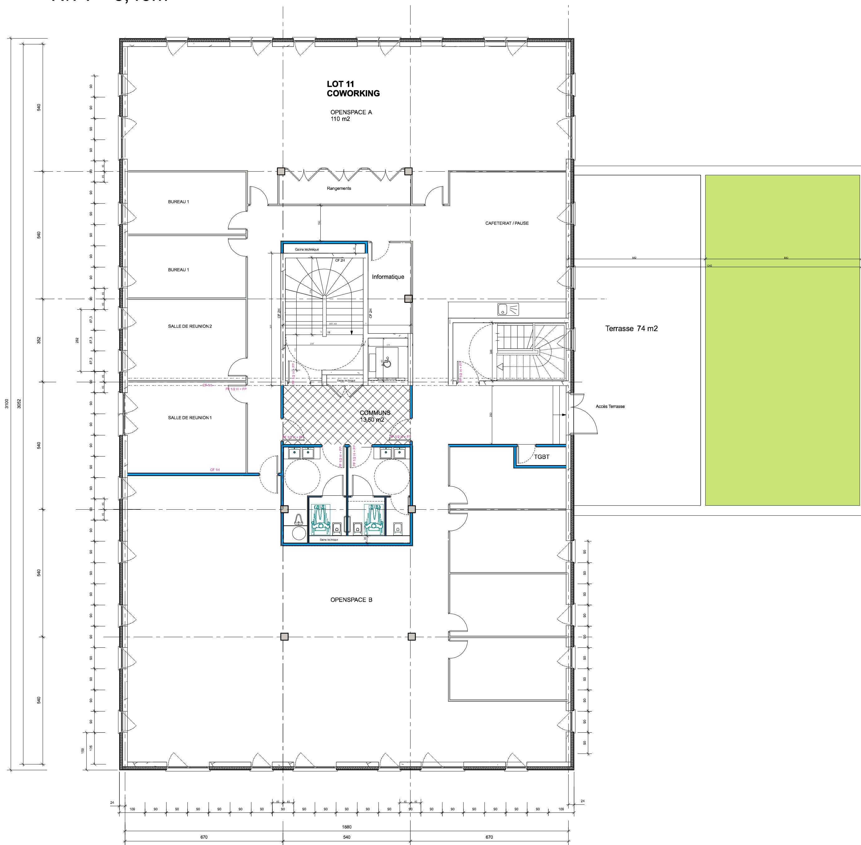
Plan étage 2 Niv : + 6,40m
