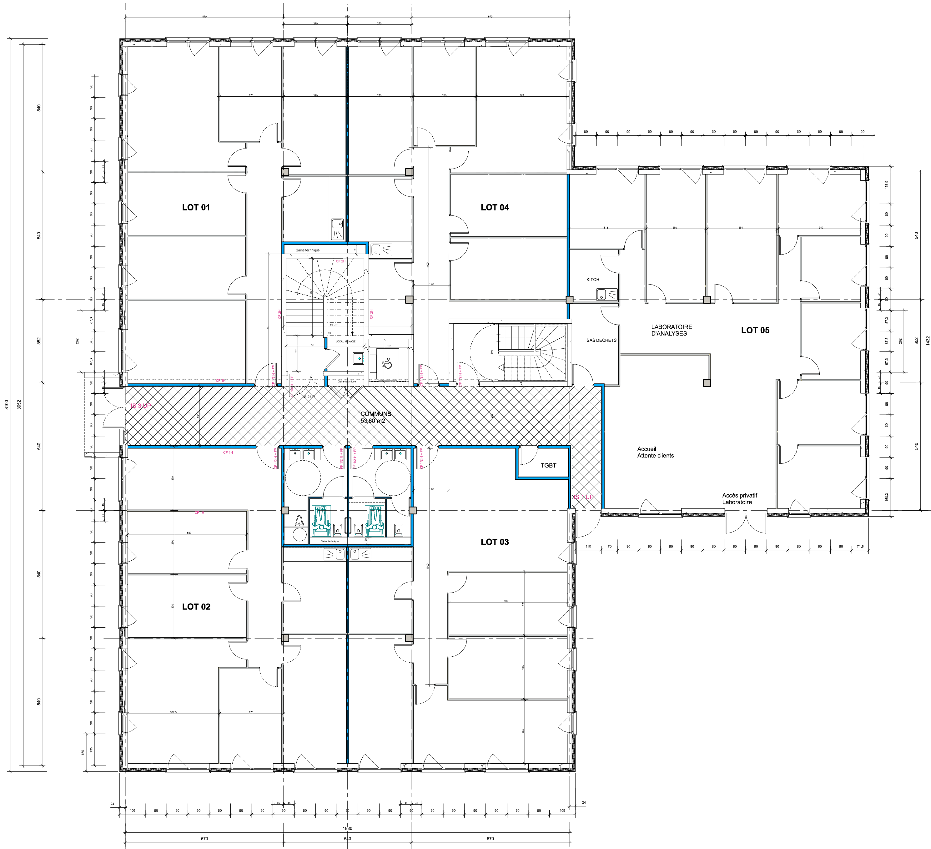
Plan étage 2 Niv : + 6,40m
