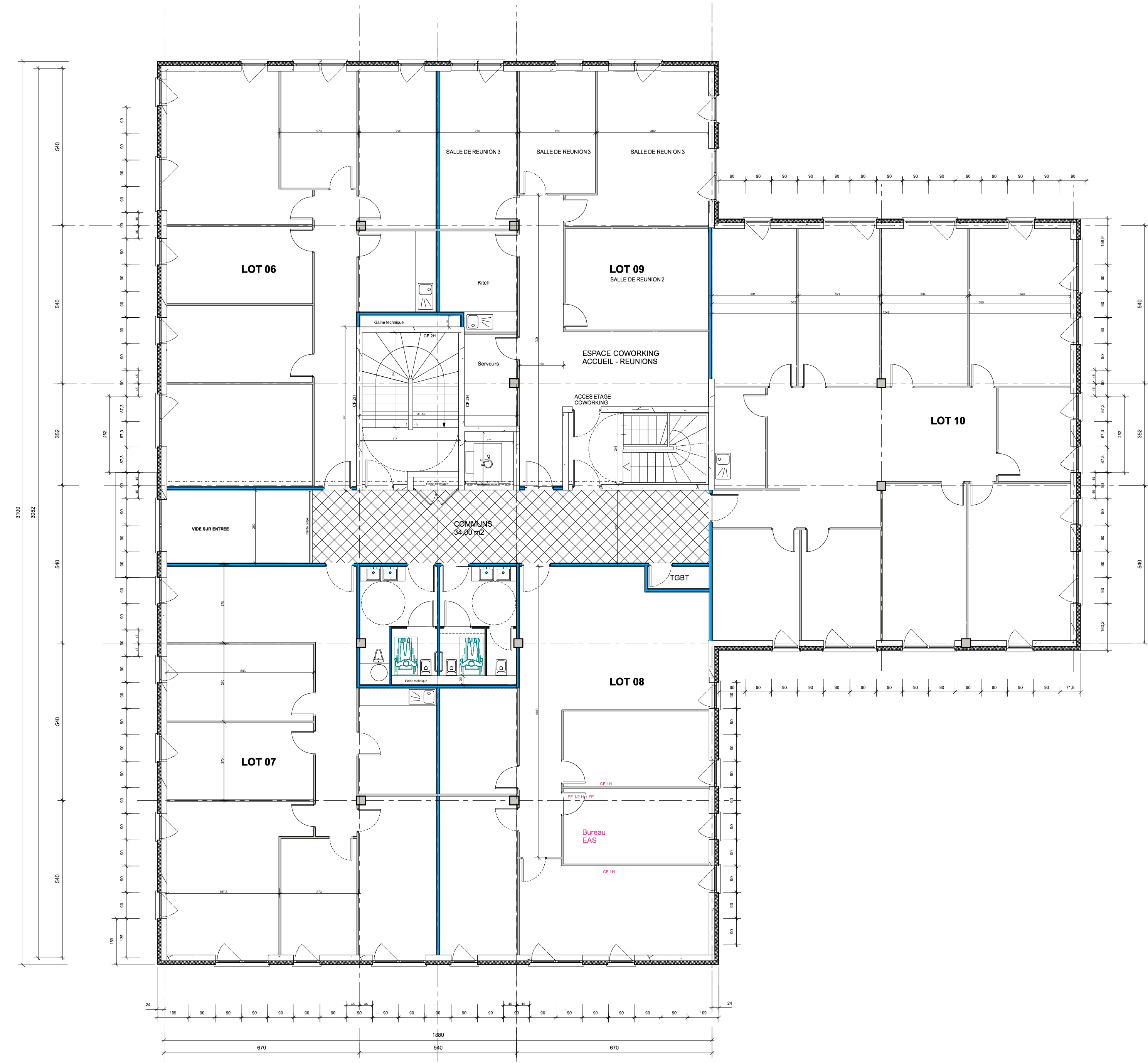
Plan étage +3 Niv : + 9,60m
